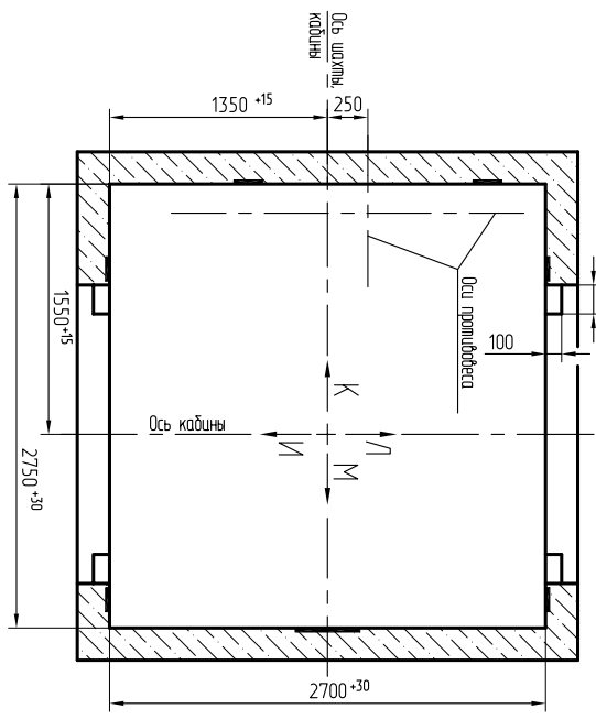
ПЛАН ШАХТЫ
